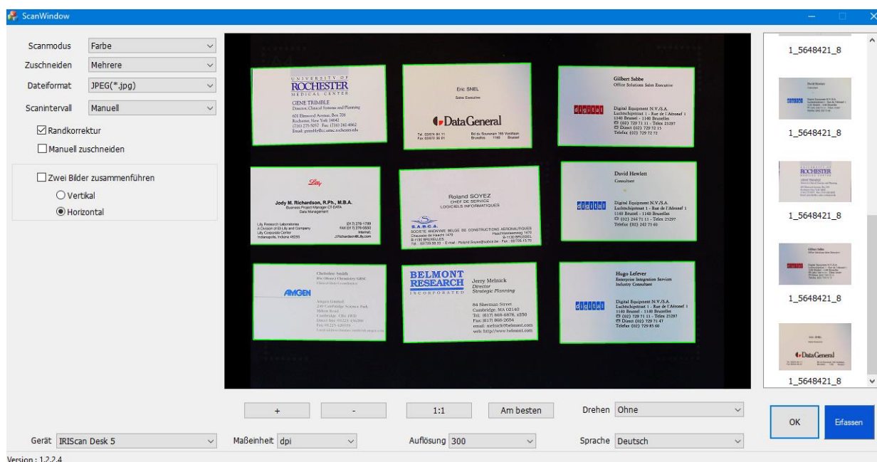
TWAIN-Benutzeroberfläche
