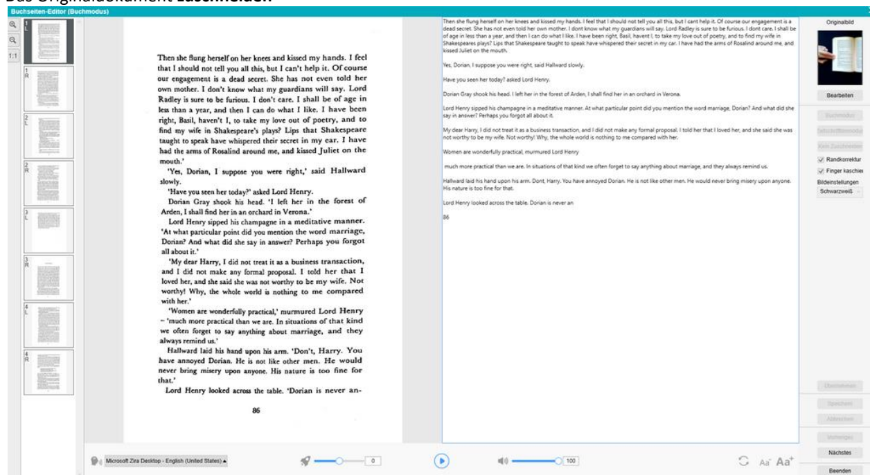
Text-in-Sprache-Editor: Vollbildansicht
