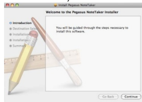
Afbeelding 1: NoteTaker-installatieprogramma
